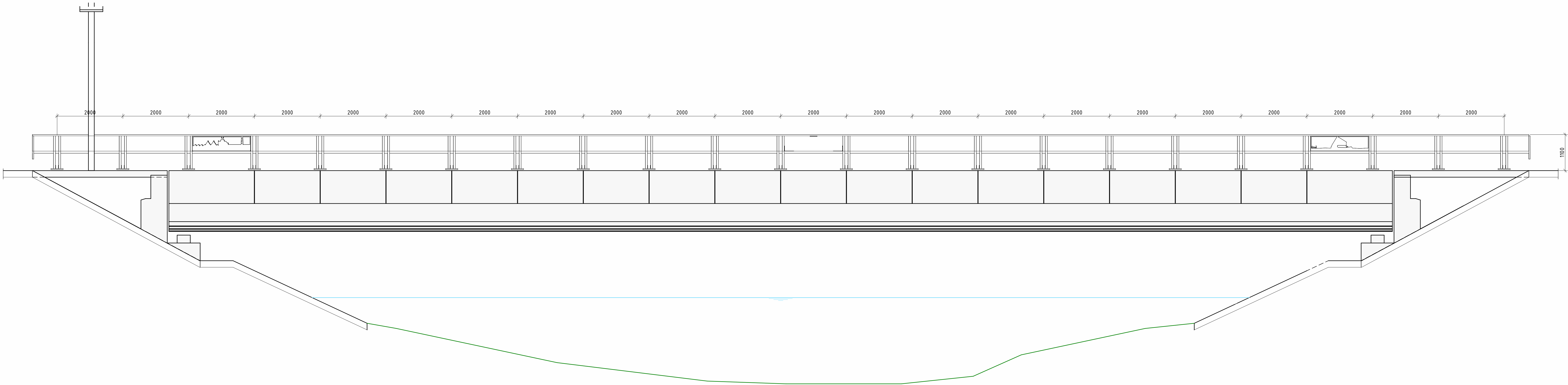
Aanzicht leuningwerk schaal 1 : 50
